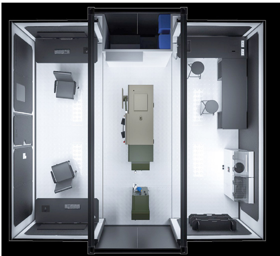
Fieldmade 3D drukas konteineru Nomad 03 iekārtojums (avots: Komersants)
